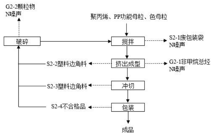
图 2.4-2 一次性餐盒生产工艺流程及产污环节图
