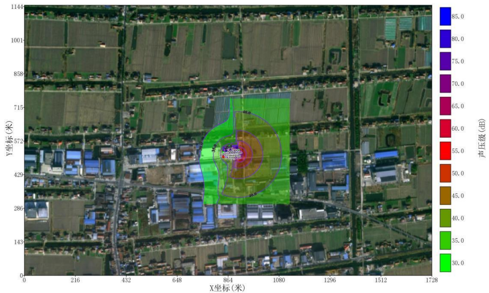
图 4.3-1 昼间噪声预测值等声级线图
