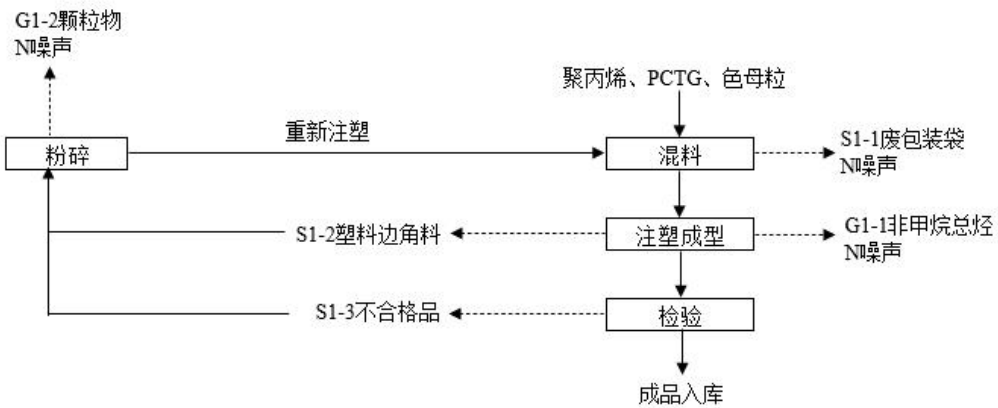
图 2.4-1 注塑件生产工艺流程及产污环节图
