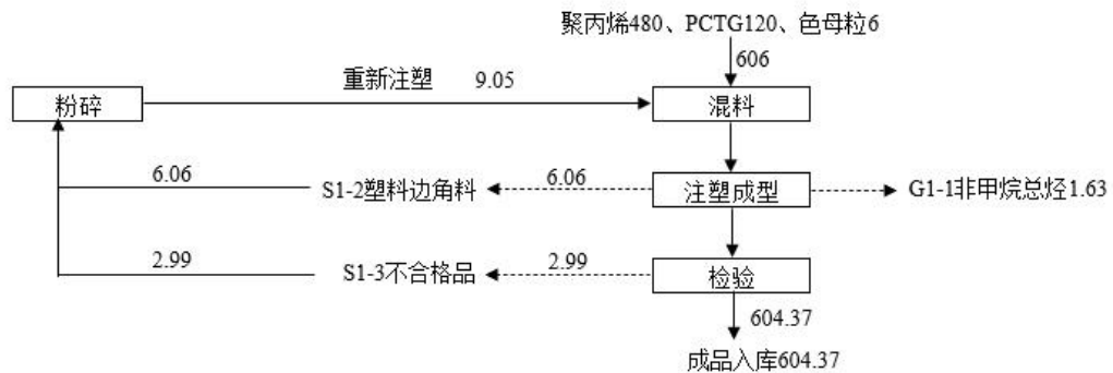
图 2.3-1 本项目注塑件生产物料平衡图（单位：t/a）
