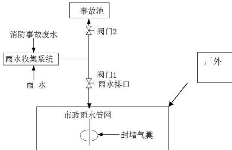
图 4.7-1 事故废水收集排放示意图
