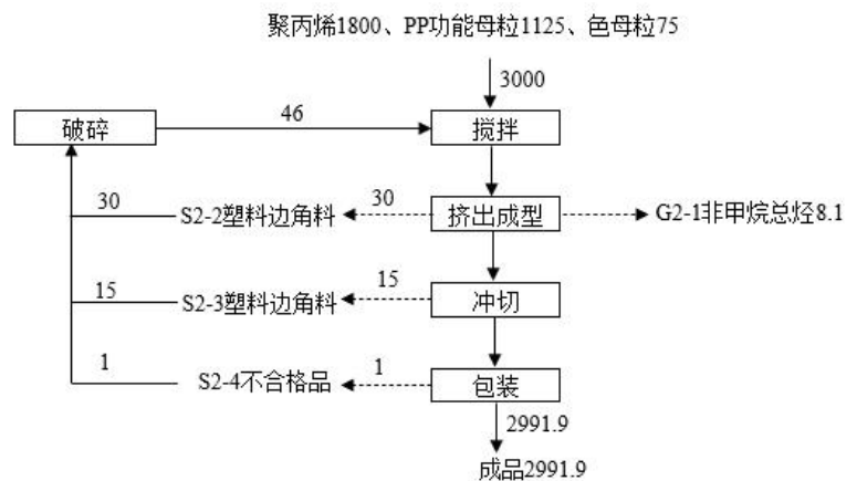
图 2.3-2 本项目一次性餐盒生产物料平衡图（单位：t/a）
